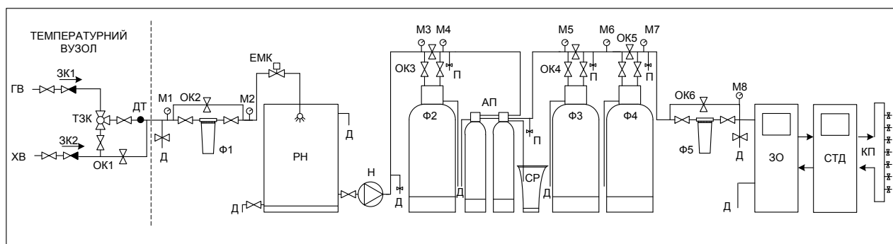
Рис. 1. Рекомендована схема побудови системи водоочиснення
